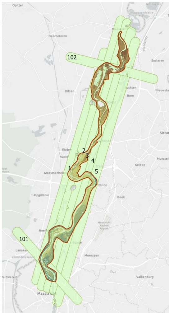
Figuur 1: AHN Special Grensmaas 2025 inclusief vliegstroke. De inwinning is uitgevoerd op 11 april 2025.
