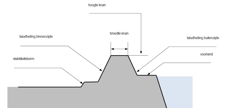
Dwarsprofieltype 3
