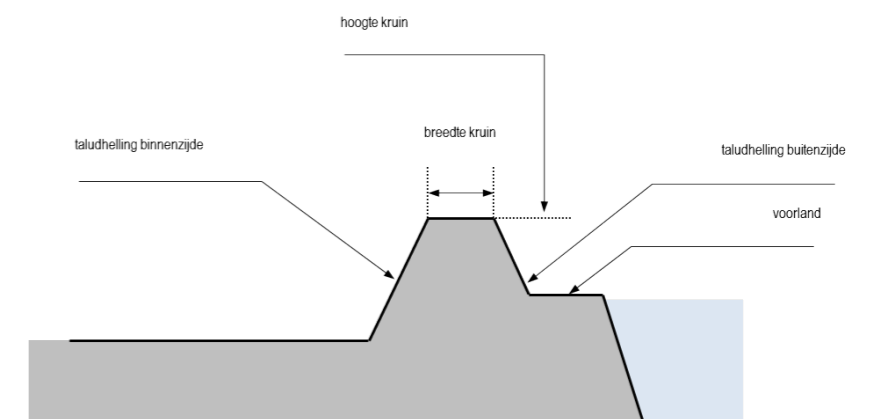
Dwarsprofieltype 4
