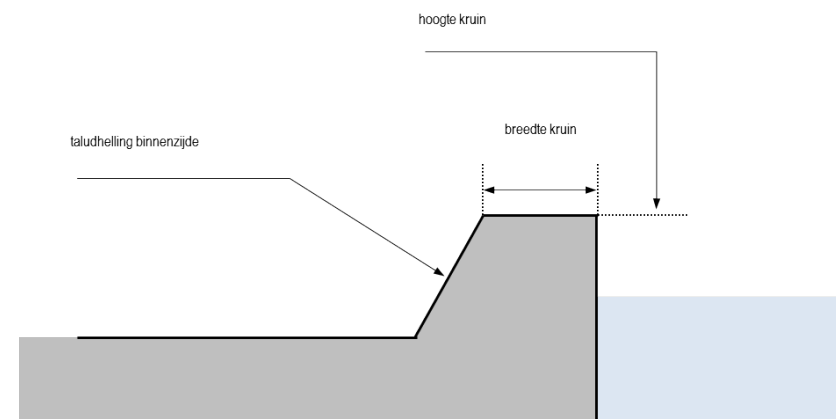
Dwarsprofieltype 5
