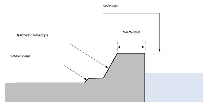
Dwarsprofieltype 6
