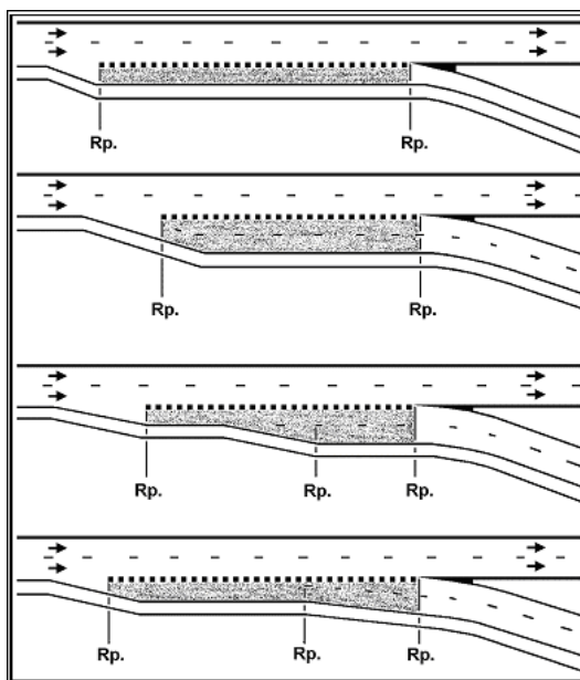
Afbeelding 91: Uitrijstroken.
