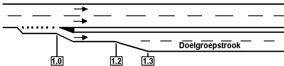
Afbeelding 26: Locatiebepaling doelgroepstrook.
