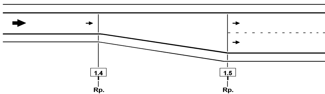
Afbeelding 106: Registratiepunt van "rijstroken" bij zachte overgang. Het aantal rijstroken verandert van 1 naar 2 tussen de registratiepunten.
