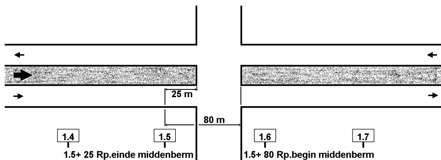
Afbeelding 157: Middenberm wordt bij een gelijkvloerse kruising en/of zijstraat onderbroken.
