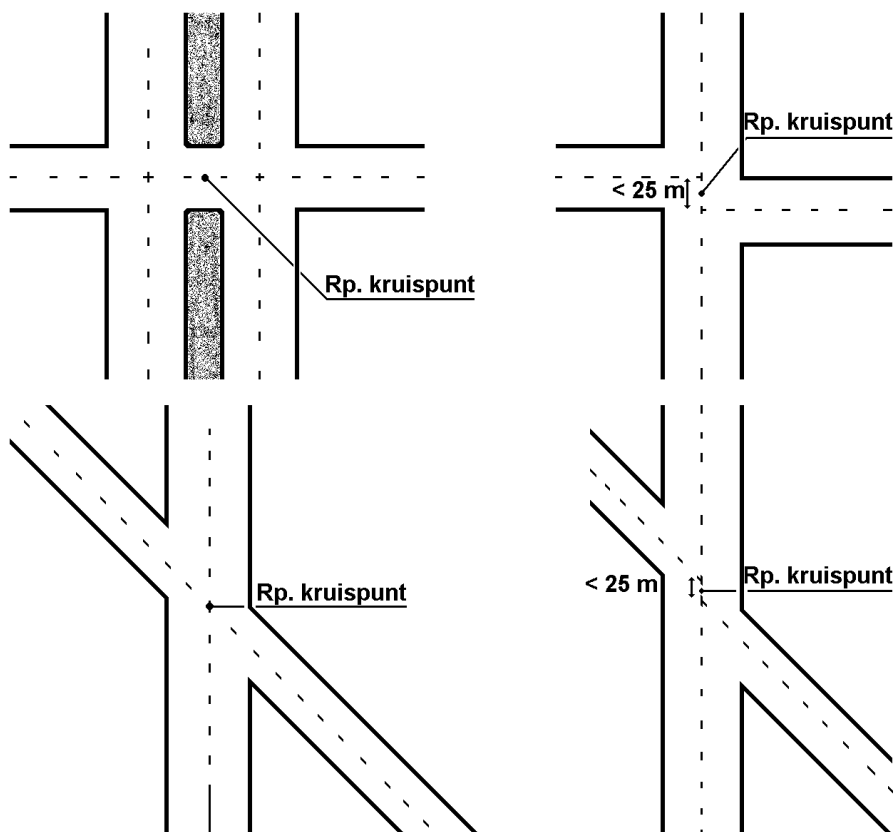
Afbeelding 62: Kruispunt varianten.
