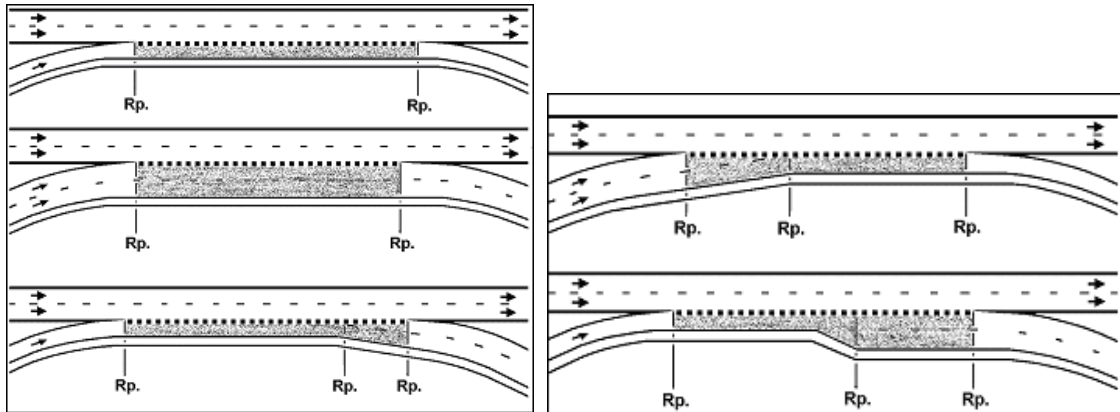
Afbeelding 94: Weefvak.
