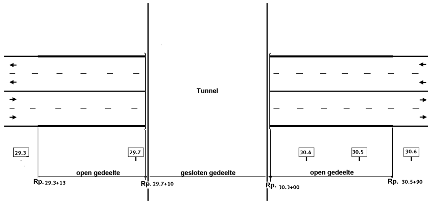
Afbeelding 54: Tunnel.
