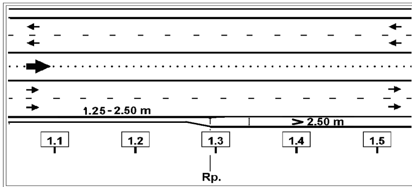
Afbeelding 44: Versmalde vluchtstrook.
