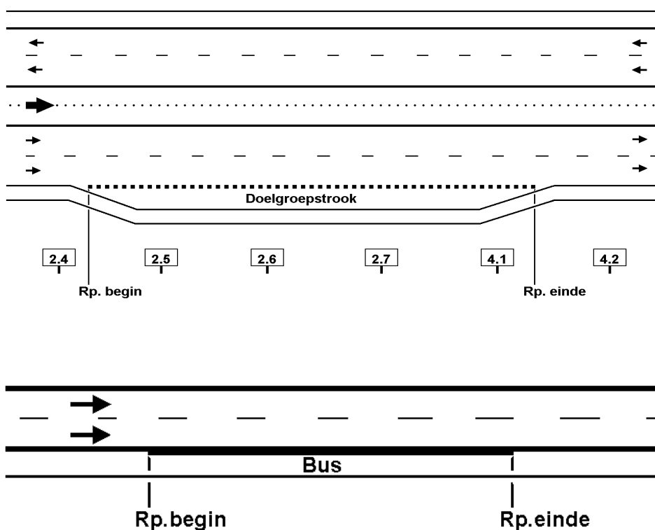
Afbeelding 25: Locatiebepaling doelgroepstrook.
