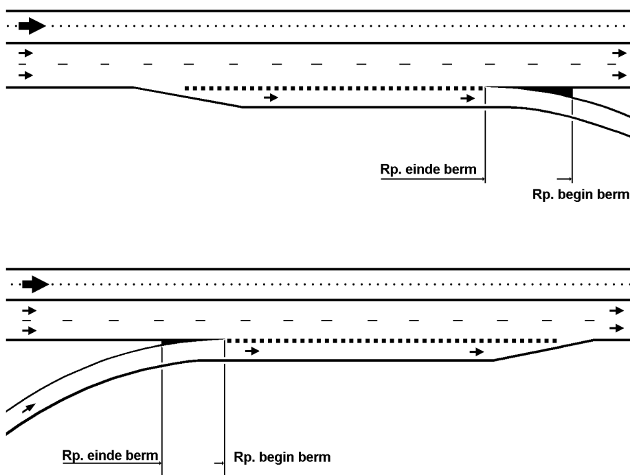
Afbeelding 149: Locatiebepaling van de buitenberm bij het puntstuk.
