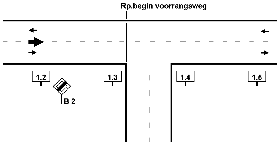
Afbeelding 144: Locatiebepaling.
