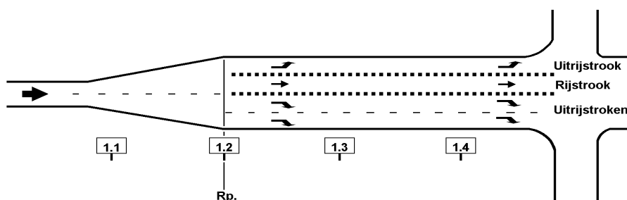
Afbeelding 117: "Rijstroken" met voorsorteervakken, een voor recht doorgaand verkeer. Bij het begin van de blokmarkering een harde overgang naar een rijstrook.
